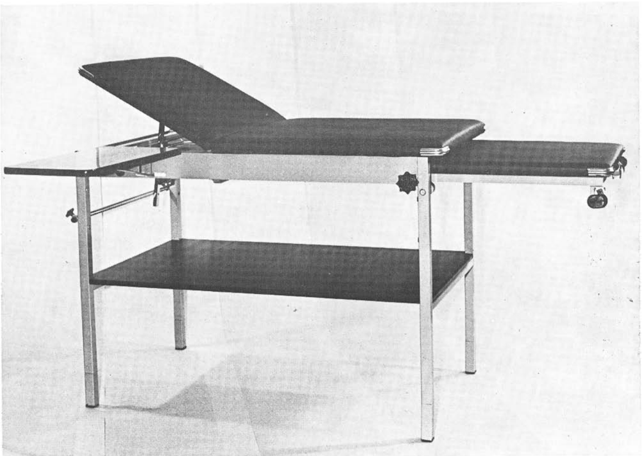
Figuur 1. De Mini-Multo N.H.G.-bank. Standaarduitvoering, aangevuld met bergplank halverwege de poten en armplank.
